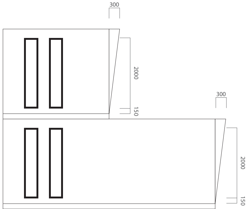
좌측면
