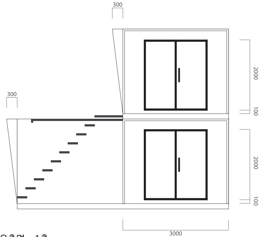
우측면 - 1층
